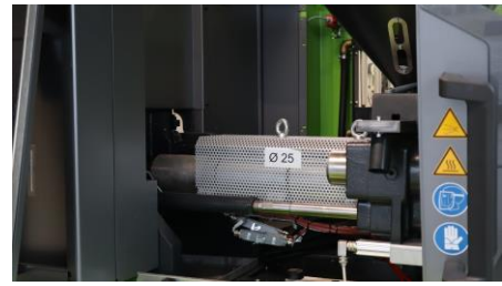
Abbildung: Plastifiziereinheit
